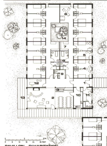
PAVILLON D'HABITATION
